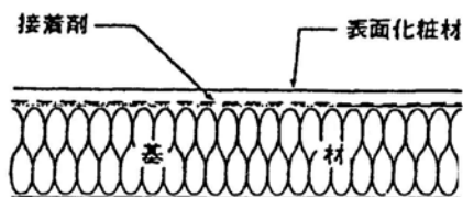
1-5 施工仕様
